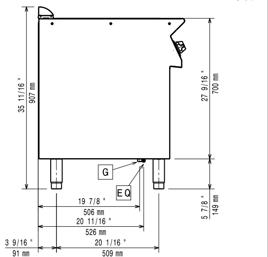
侧视
